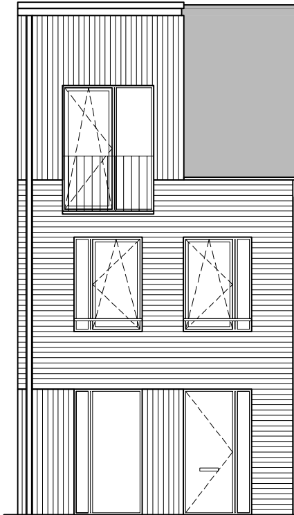
voorgevel
