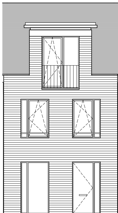
voorgevel
